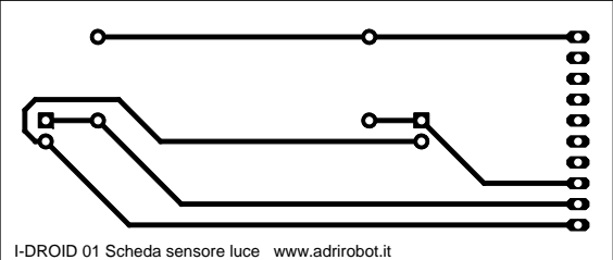
I-DROID 01 Scheda sensore luce www.adrirobot.it
