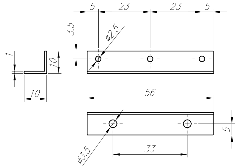
2 x Profilo alluminio 10x10x1 I=56
