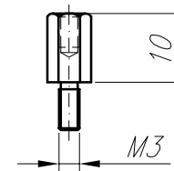
Distanziali esagonali M3x10 Qta' 8
